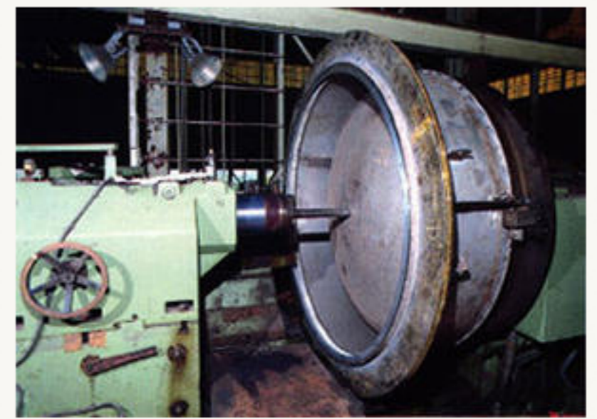
▲正面旋盤
